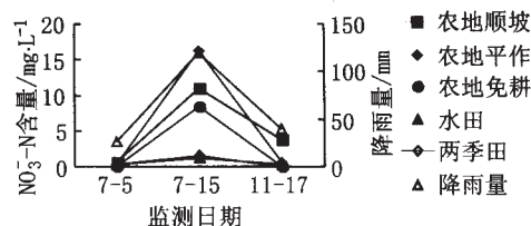
图 1 降雨与农田径流水 NO 3 - -N 含量
