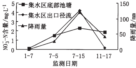
图 2 降雨与集水区径流NO 3 - -N 含量变化
