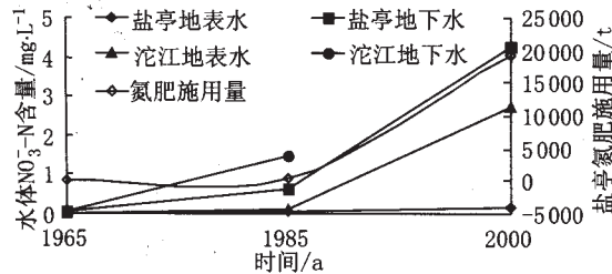
图 4 盐亭、沱江水体NO 3 - -N 含量与施肥
