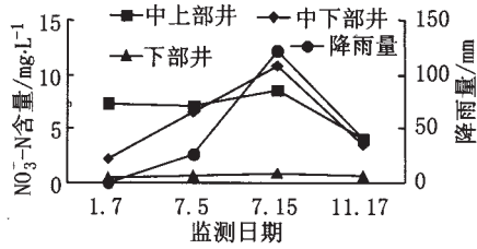
图 3 降雨与地下水NO 3 - -N 含量变化
