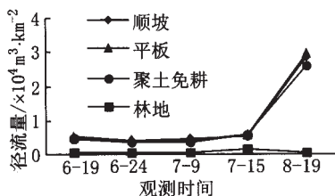
图 8 不同耕作方式耕地径流量
